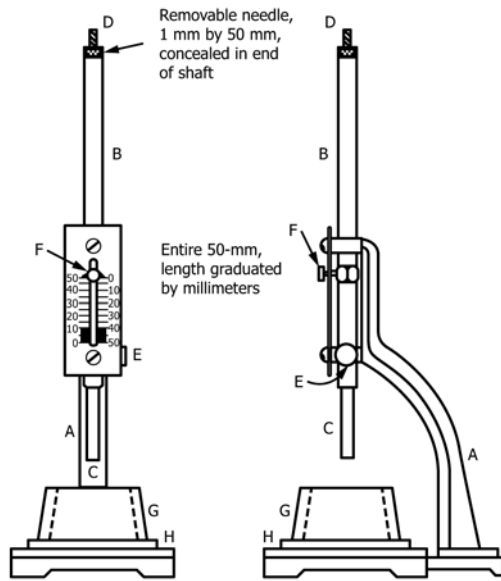
FIG. 1 Vicat Apparatus
